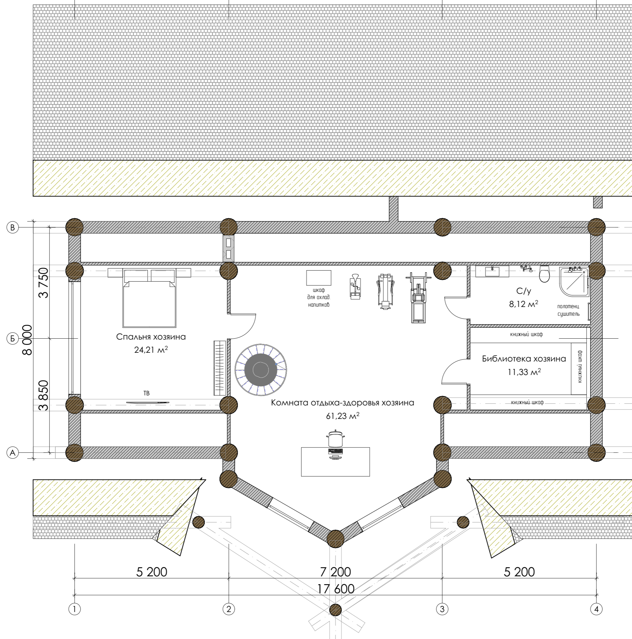
План мансарды дома
